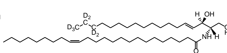
C24:1 Ceramide-d7 (d18:1-d7/24:1)
